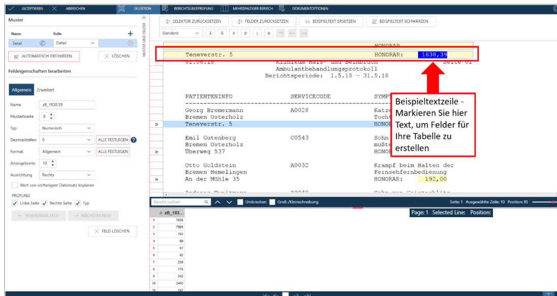
Abbildung 4-21: Felder hervorheben.
