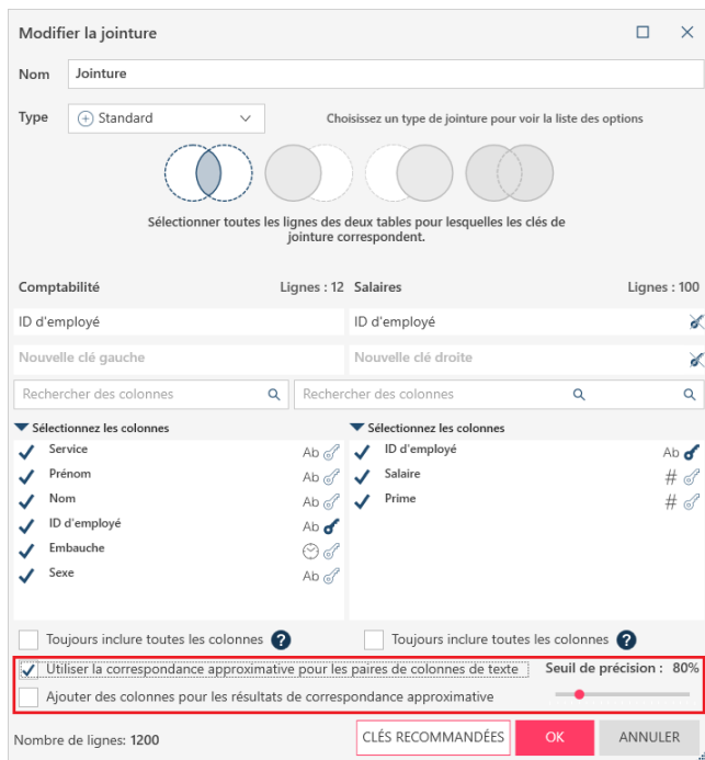
Figure 4-46. Correspondance approximative activée dans la boîte de dialogue Configuration de jointure.
