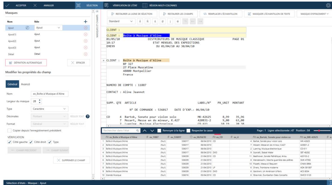
Figure 2-19. Fenêtre Conception de l'état de Data Prep Studio.
