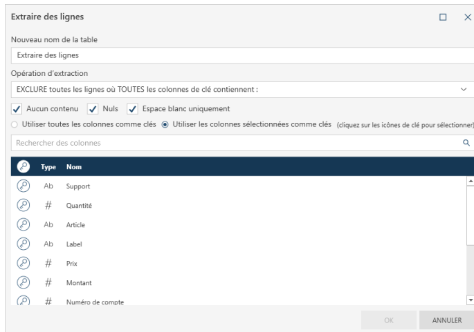
Figure 4-70. Boîte de dialogue Extraire des lignes.
