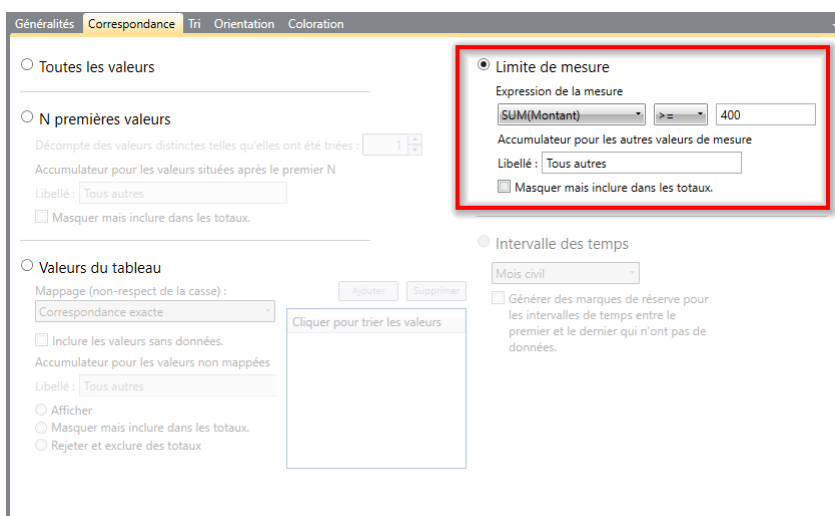
Figure 16-16. Spécification des limites de récapitulatif.
