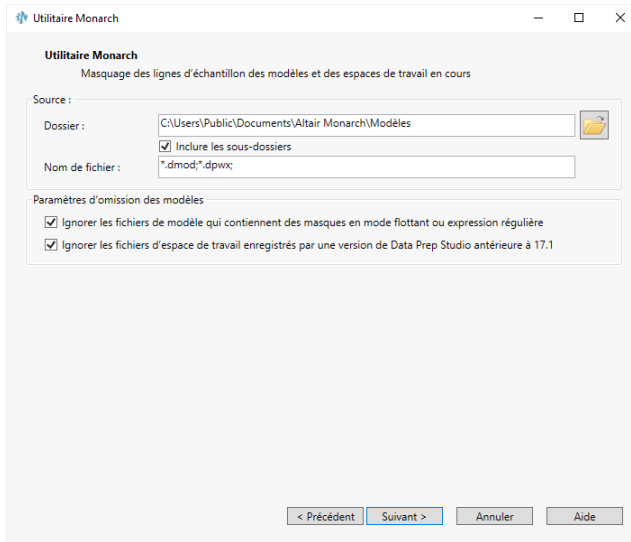
Figure 23-28. Spécification des paramètres d'omission des modèles.
