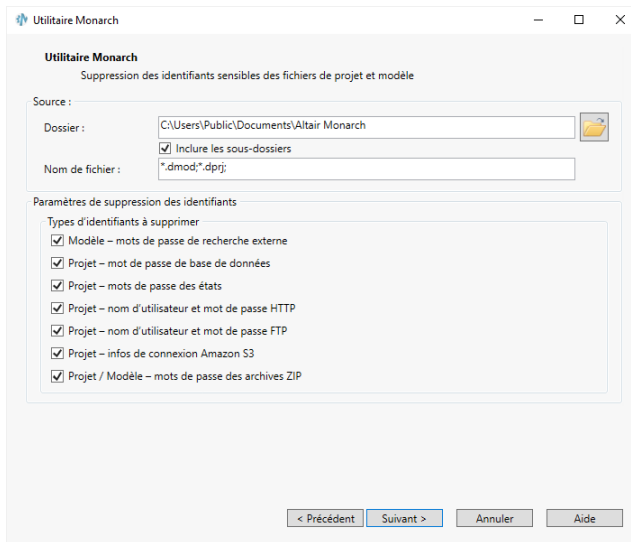
Figure 23-34. Spécification des identifiants à supprimer des projets et des modèles.
