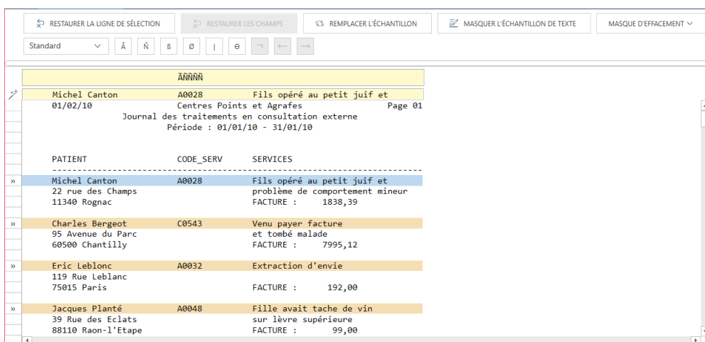
Figure 4-26. Les lignes se sélectionnent si elles contiennent des données correspondant aux caractères de sélection indiqués.
