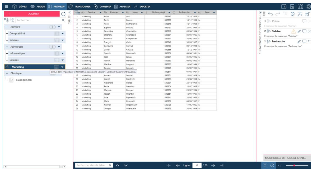
Figure 4-86. Liste de changements de la table Jointure (Comptabilité + Salaires) déplacée vers la table Marketing .
