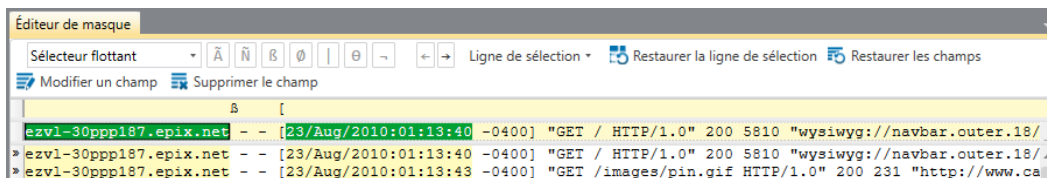
Figure 8-23. Sélecteur flottant avec caractère de sélection blanc.
