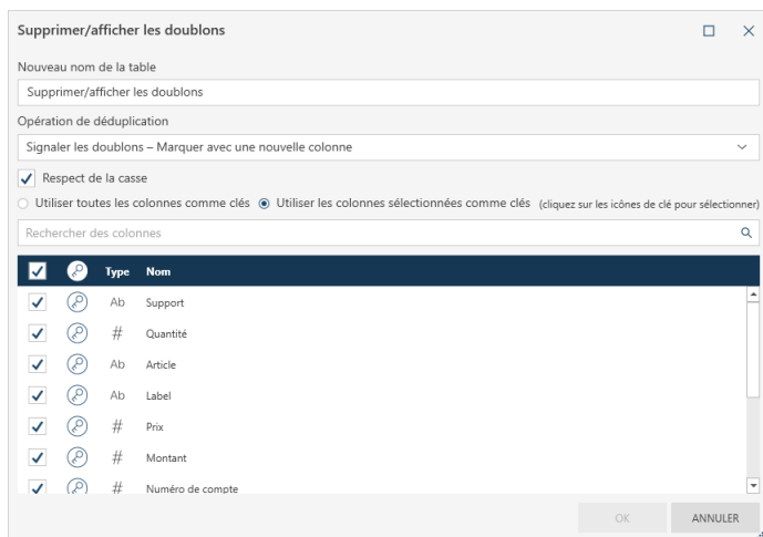
Figure 4-69. Boîte de dialogue Supprimer/afficher les doublons.
