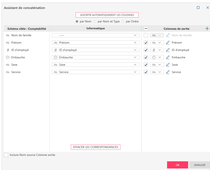
Figure 4-52. Boîte de dialogue Assistant de concaténation.
